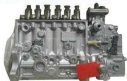
PC360-7小松 0402066729 高压油泵
