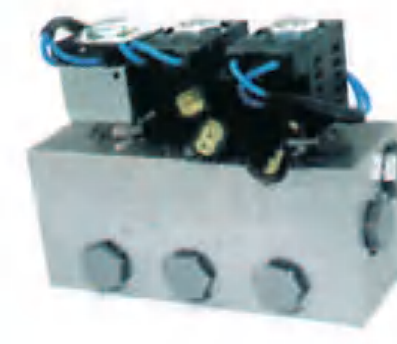
油源阀块总成
